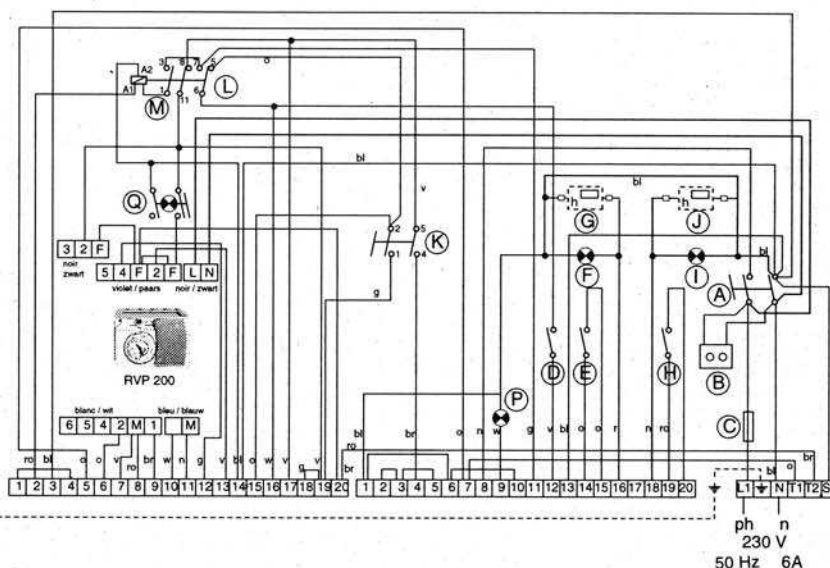
Principeschema
